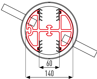
PROFIL ROND DU SYSTÈME 50 (monté dans une douille de sol)
