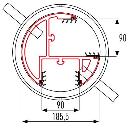
PROFIL ROND 90° DU SYSTÈME 80
