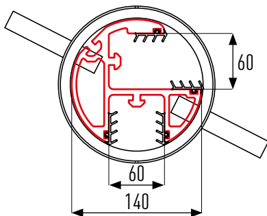
PROFIL ROND 90° DU SYSTÈME 50
