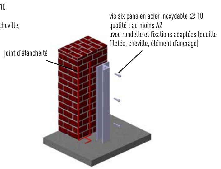
MONTAGE DU PROFIL EN APPLIQUE
