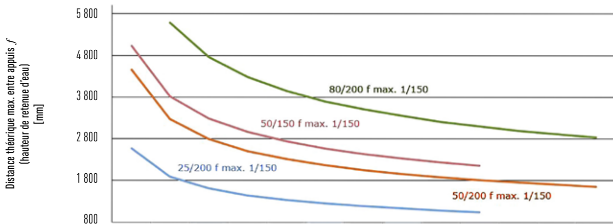
Distance théorique entre appuis en fonction de la flèche max. f (hauteur de retenue d'eau)
