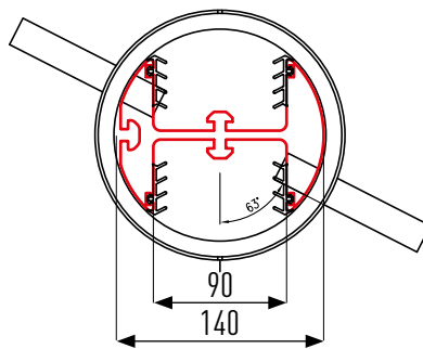
PETIT PROFIL ROND DU SYSTÈME 80 (monté dans une douille de sol)
