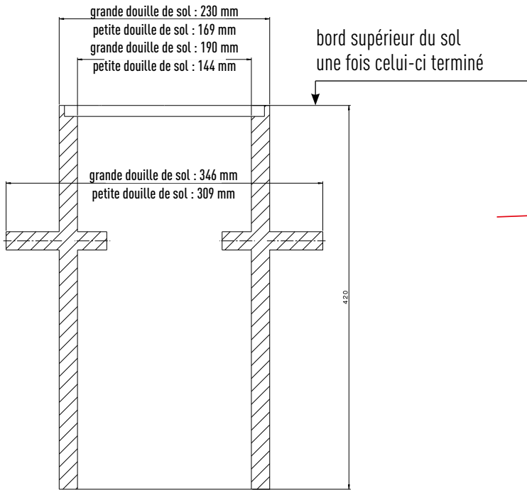
DOUILLE DE SOL
