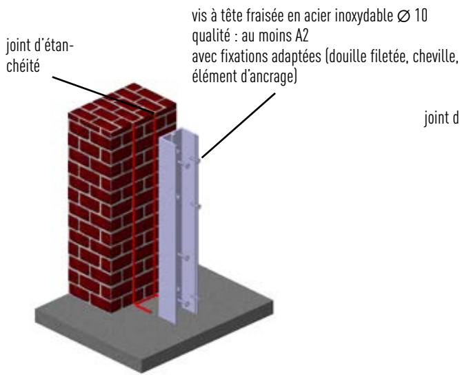
MONTAGE DU PROFIL EN U
