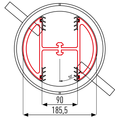
GRAND PROFIL ROND DU SYSTÈME 80 50 et 80 Vario (monté dans une douille de sol)
