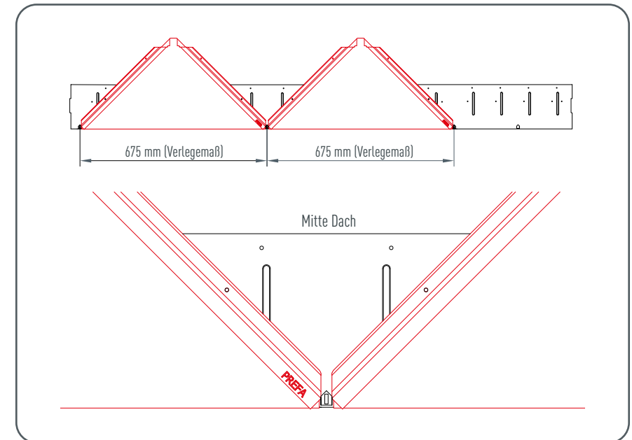
Abbildung 63 • Saumstreifen – Besonderheiten bei Wandraute 44 × 44
