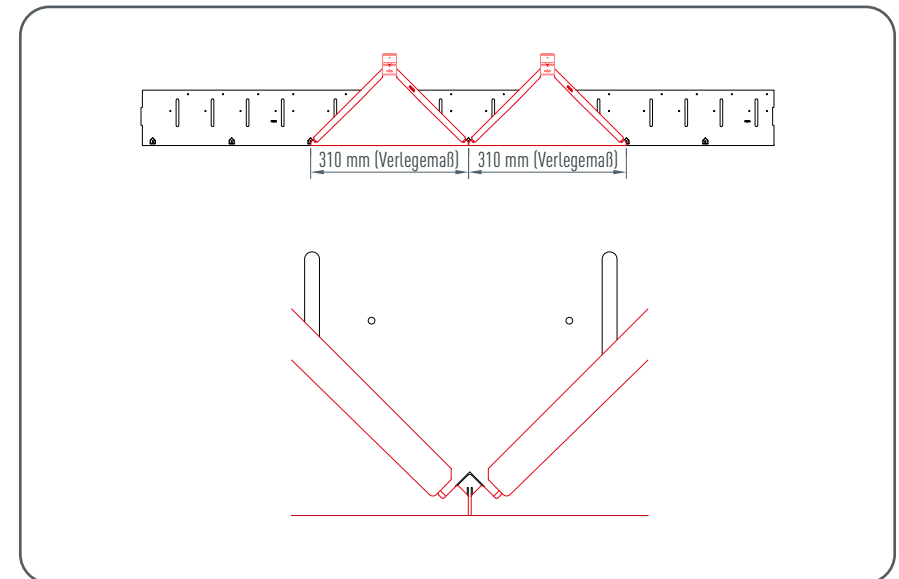
Abbildung 21 · Wandraute 20 × 20 – Startplatte
