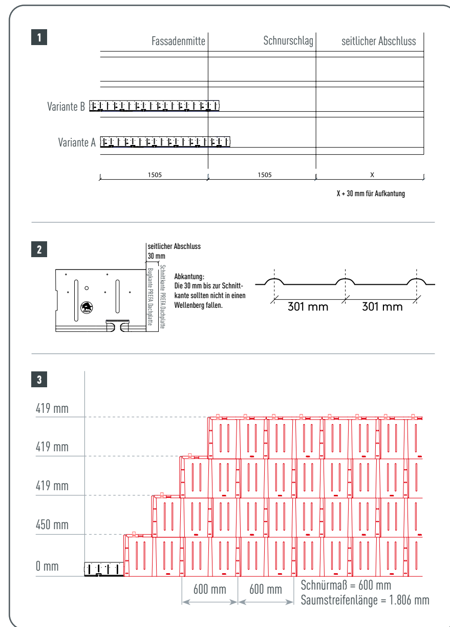
Abbildung 45 · Dachplatte – Schnürmaß
