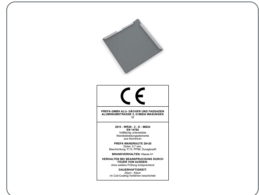
Abbildung 19 · Wandraute 20 × 20
