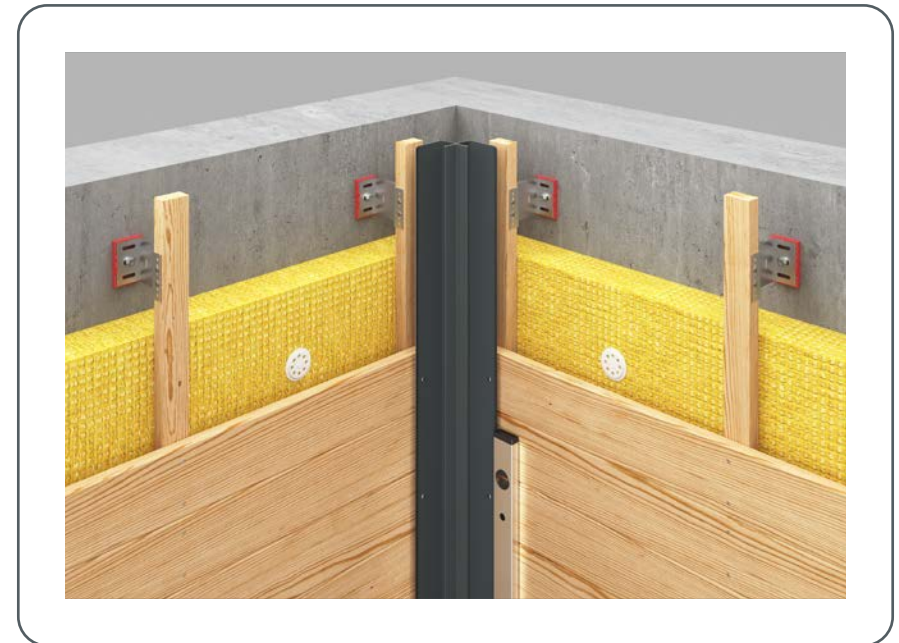
Abbildung 65 • Innenecke – PREFA Kleinformat
