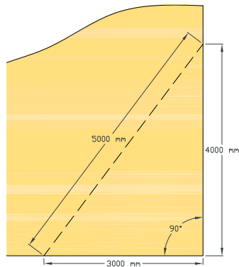
Abbildung 2 · Schnürung
