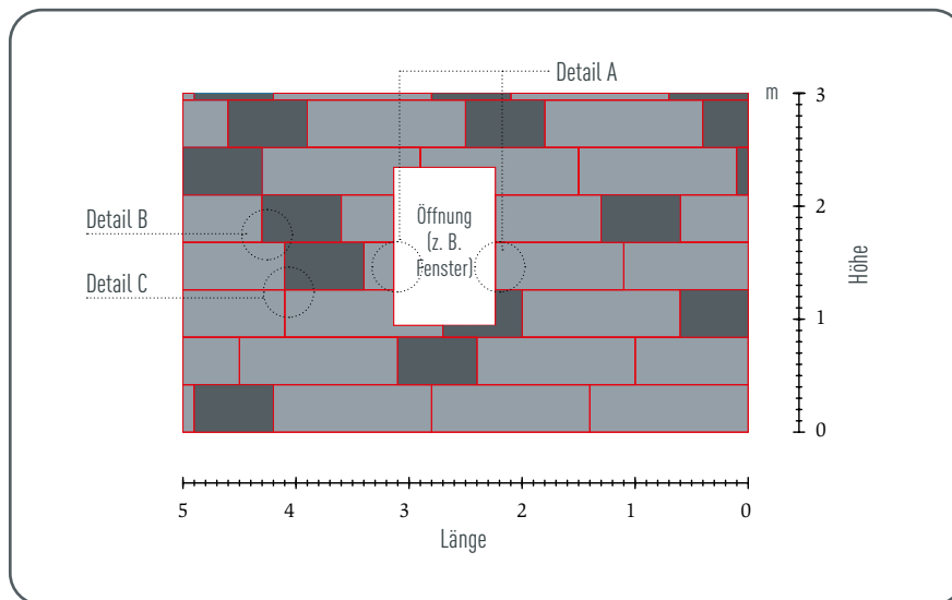
Abbildung 37 · Fassadenpaneel FX.12 – Beispiel einer falschen Verlegung
