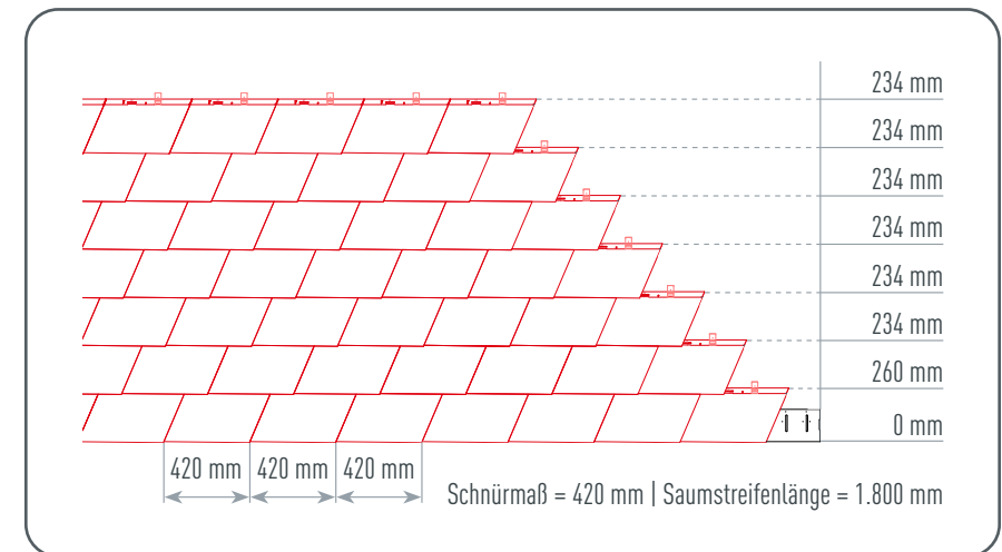
Abbildung 8 · Wandschindel – Schnürmaß
