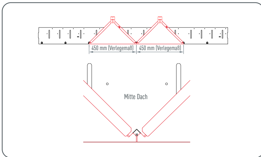
Abbildung 62 • Saumstreifen – Besonderheiten bei Wandraute 29 × 29
