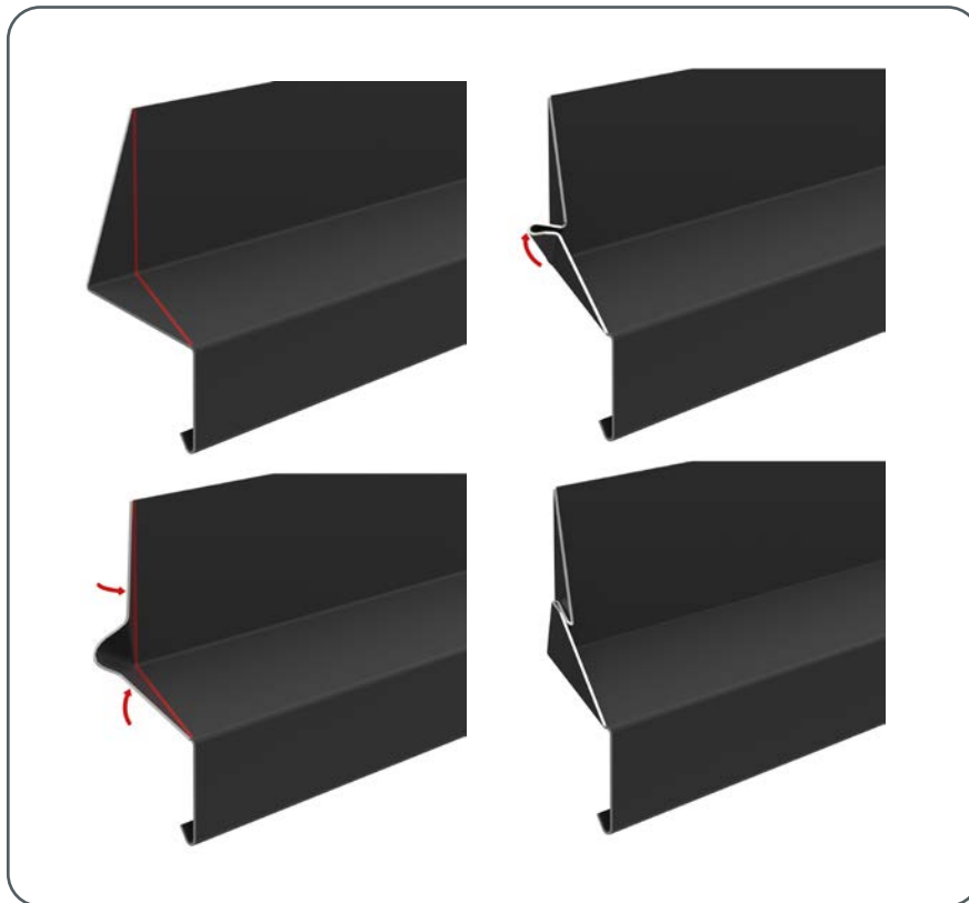
Abbildung 81 · Wetterschenkel Fenstersturz
