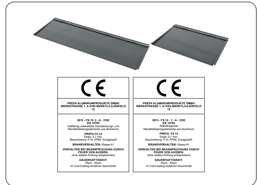
Abbildung 33 • Fassadepaneel FX.12
