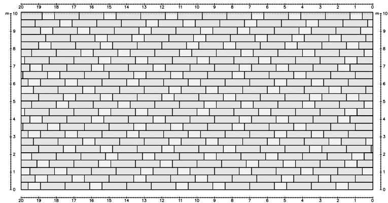
Abbildung 40 - Fassadenpaneel FX.12 - Verlegebeispiel Variante 3
