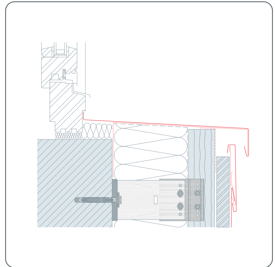
Abbildung 86 · Fensterbank
