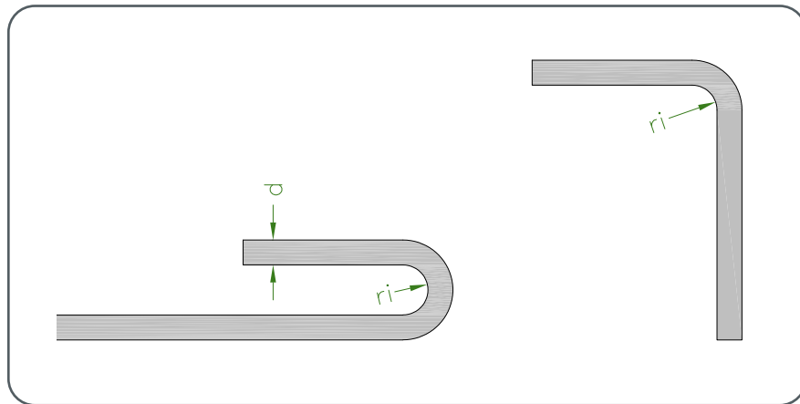
Abbildung 3 • Ergänzungsbänder Biegeradius
