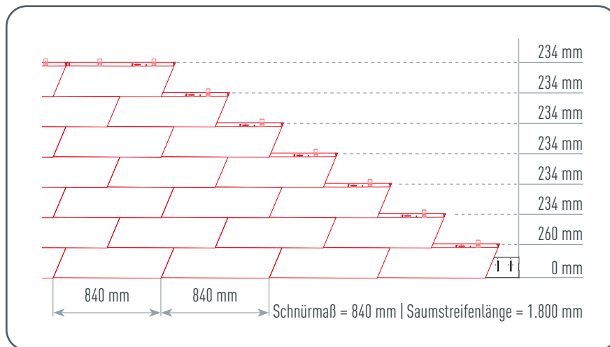
Abbildung 9 • Wandschindel XL – Schnürmaß
