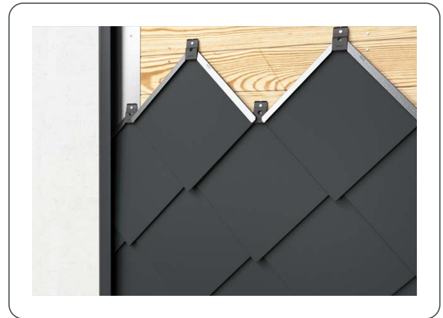
Abbildung 71 • Seitlicher Anschluss
