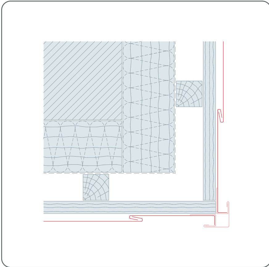
Abbildung 68 • Außenecke – PREFA Kleinformat
