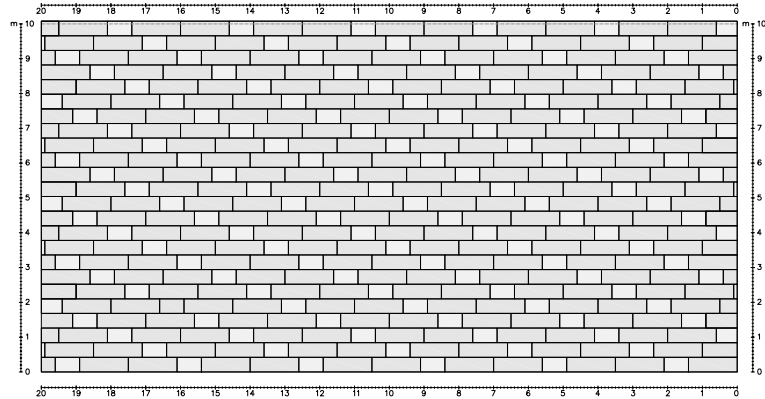
Abbildung 39 - Fassadenpaneel FX.12 - Verlegebeispiel Variante 2
