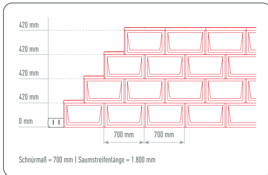
Abbildung 49 • Dachplatte R.16 – Schnürmaß
