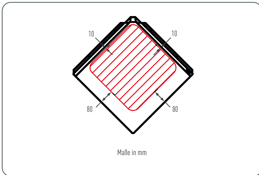
Abbildung 32 · Wandraute 44 × 44 – Montagebereich
