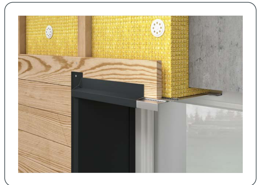
Abbildung 82 · Montage Wetterschenkel Fenstersturz
