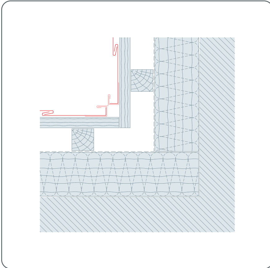
Abbildung 66 • Innenecke – PREFA Kleinformat
