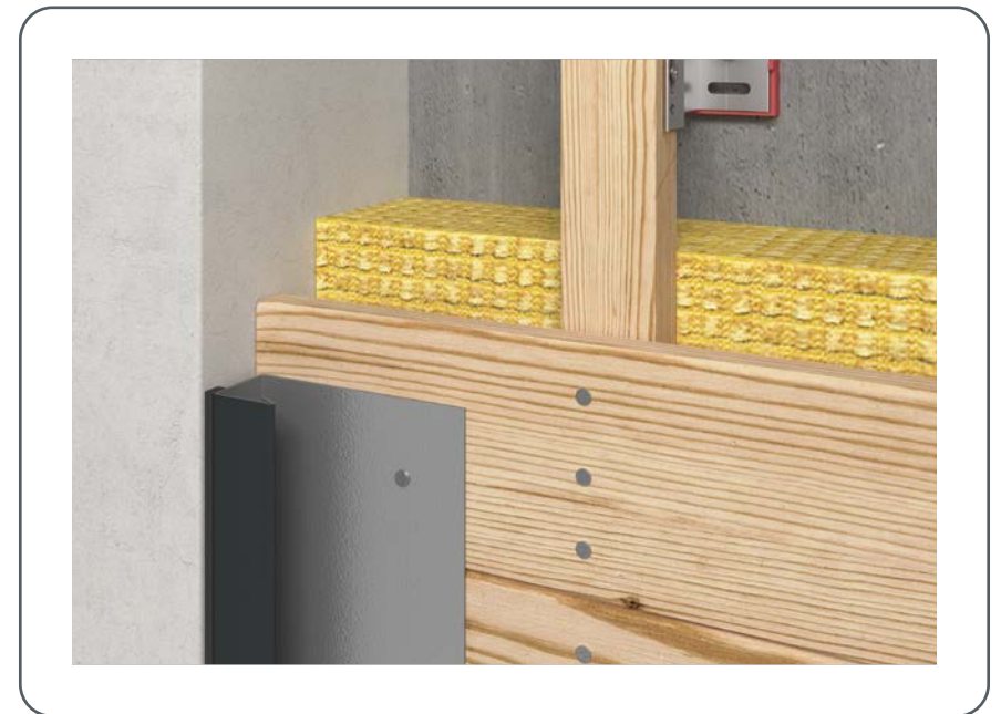
Abbildung 69 • Seitlicher Anschluss – Vorbereitung
