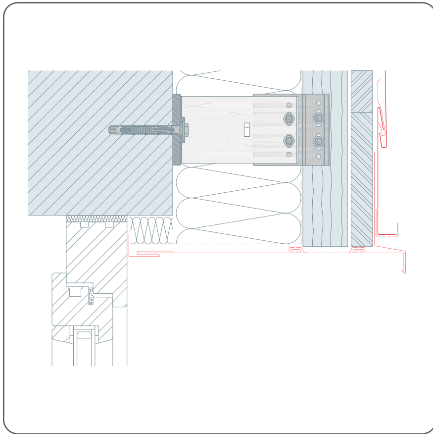
Abbildung 85 · Fenstersturz
