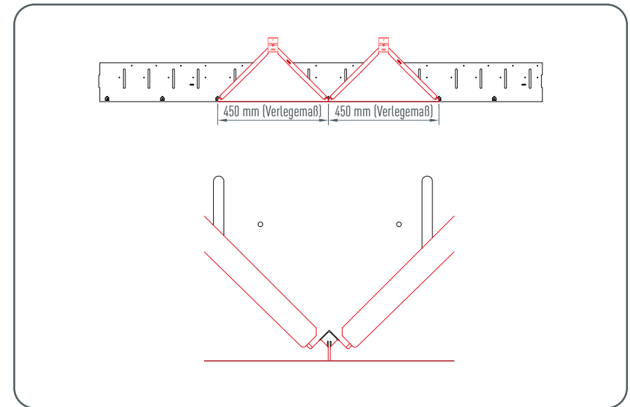
Abbildung 25 · Wandraute 29 × 29 – Markierung Saumstreifen
