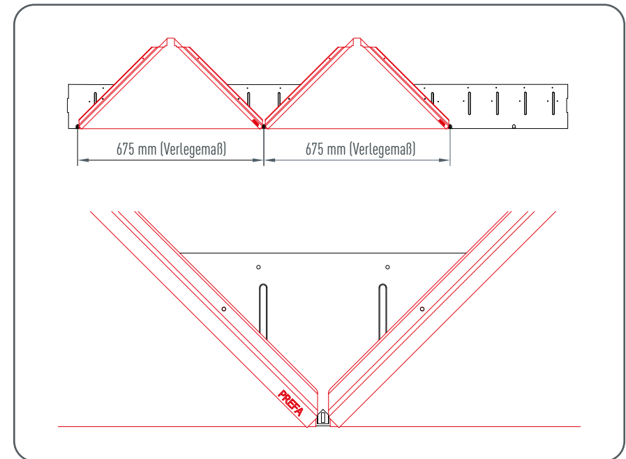
Abbildung 30 · Wandraute 44 × 44 – Markierung Saumstreifen
